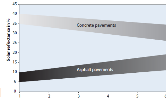
Reflectividad solar del asfalto convencional y el hormigón
