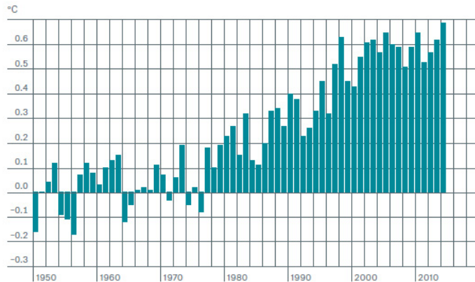
Desviaciones de la temperatura anual respecto de la media del periodo 1901-2000. Fuente: Munich Re con datos de NCDC y NOAA de Estados Unidos.
